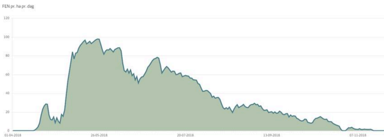
Figur 3. Den beregnede daglige græsvækst i 2018 uden korrektion for vandbalance
