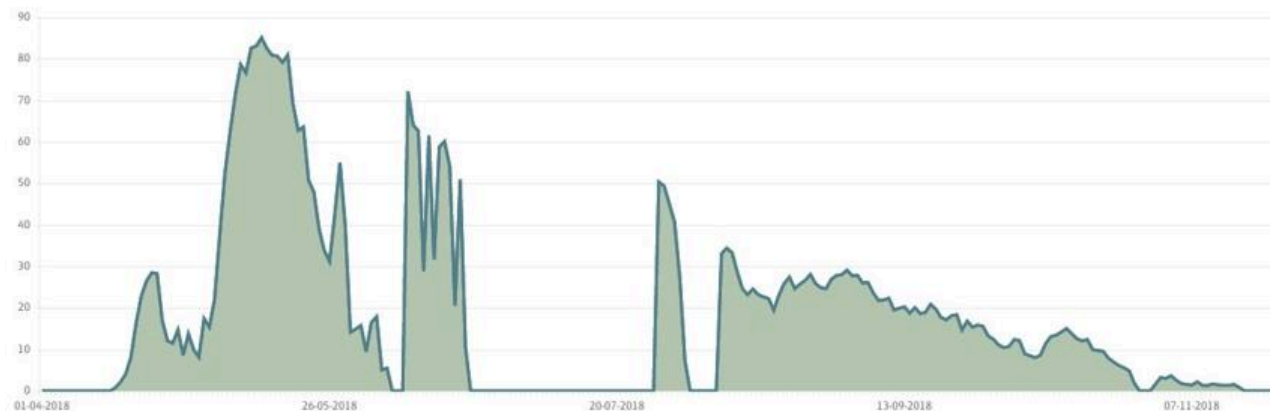
Figur 4. Den beregnede daglige græsvækst i 2018 med korrektion for vandbalance
