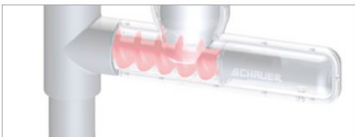
Billede 1: Princippet til placering af den lille snegl og motor mellem foderkassen (øver sneglen) og ned-faldetret til krybben til venstre (illustration: BoPill)
