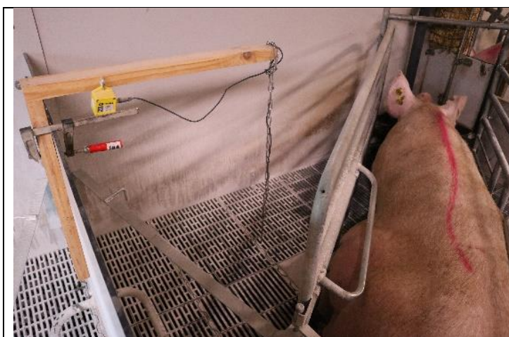
Figur 5. Føler til måling af temperatur i farestien med logger.
