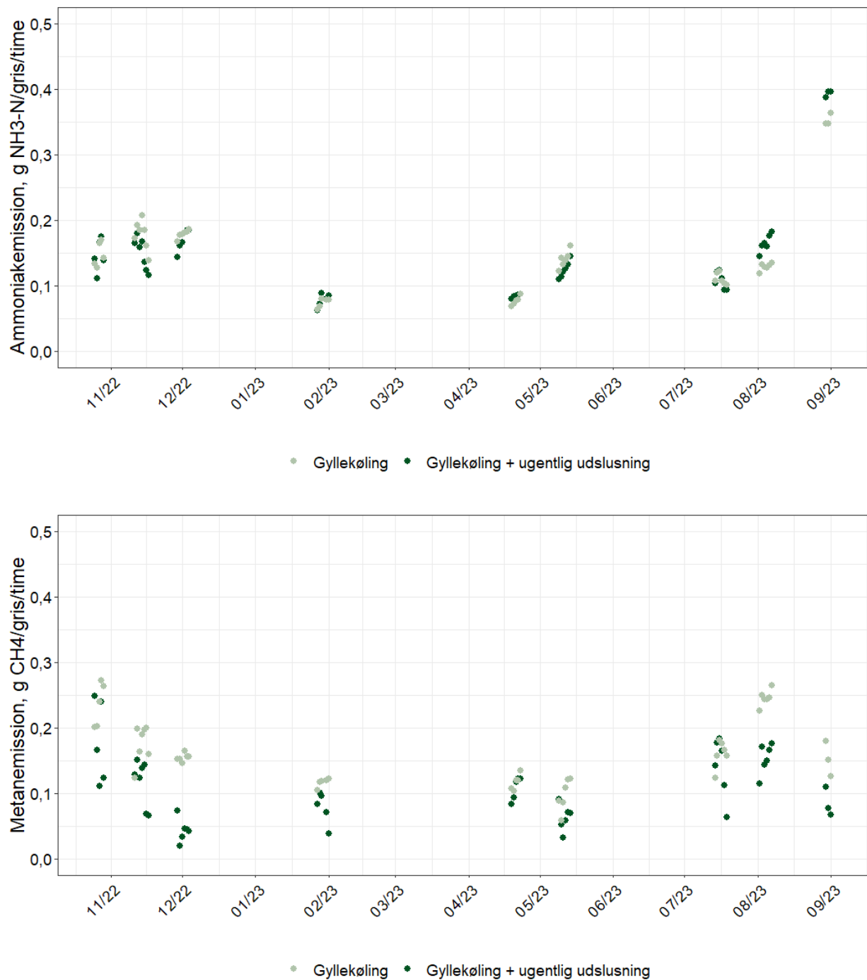
Figur 3A. Ammoniak-, metan og lugtemission ved gyllekøling sammenlignet med gyllekøling kombineret med ugentlig udslusning på enkelte måledage.
