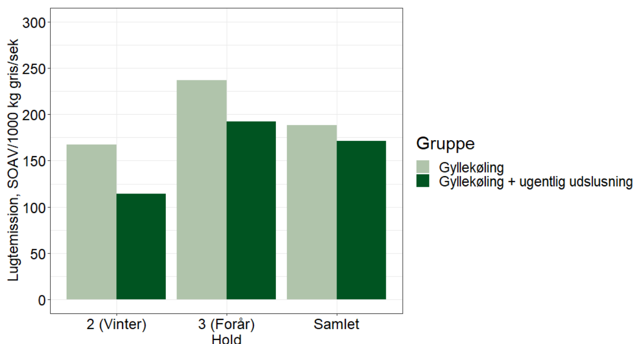
Figur 5. Lugtemission ved gyllekøling sammenlignet med gyllekøling kombineret med ugentlig udslusning for hvert af de to hold (5 måledage for Hold 2; 11 måledage for Hold 3), samt den samlede lugtemission for de to hold.
